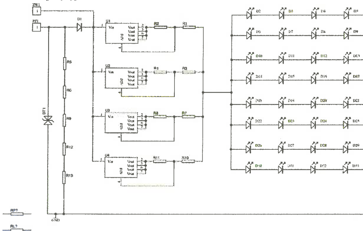
Rys. 5: Schemat połączeń dla światła pozycyjnego lamp HOR 124
