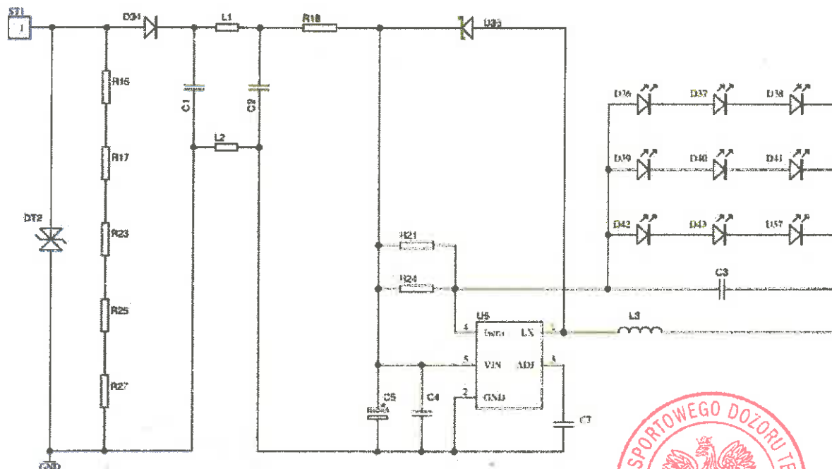
Rys. 6: Schemat połączeń dla światła hamowania lamp HOR 124
