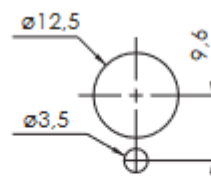
Foratura pannello Drilling mask
